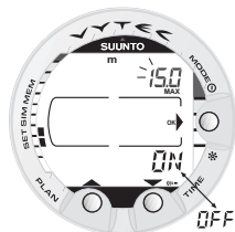
Bild 4.27. Inställning av djuplarm. Tryck på scroll-knapparna för att aktivera/inaktivera larmet och ställa in maxdjupet.
