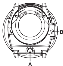
Bild 2.3. Djupsensor (A), vatten-/dataöverföringskontakter (B).
