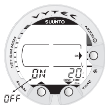
Bild 4.26. Inställning av dyktidslarm. Tryck på scroll-knapparna för att aktivera/inaktivera larmet och ställa in dyktiden.
