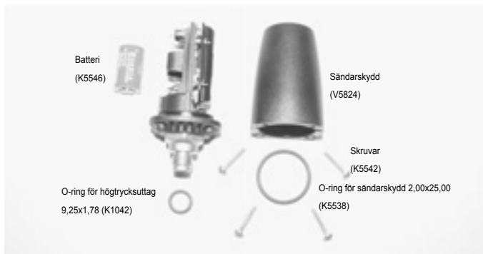
Bild 5.3. Den trådlösa sändarens delar. Koden står för reservdelsnumret.
