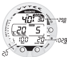
Bild 3.14. Obligatoriskt säkerhetsstopp. Du ska göra ett obligatoriskt säkerhetsstopp i djupintervallet mellan 6 och 3 meter. Om du trycker på TIME visas den alternativa displayen.
