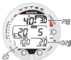
Abb. 3.14. Verbindlicher Sicherheitsstopp. Sie werden aufgefordert, einen verbindlichen Sicherheitsstopp in einem Tiefenbereich zwischen 6m und 3m [20 Fuss – 10 Fuss] durchzuführen. Durch Drücken von TIME erscheint die alternative Anzeige.
