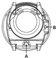
Figuur 4.10. Dieptesensor (A), watercontact voor gegevensoverdracht (B)
