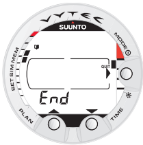
Fig. 4.12. Logboek, einde van het geheugen. De tekst 'END' wordt tussen de oudste en meest recente duik in getoond.
