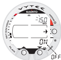
Fig. 4.27. Het instellen van het diepte-alarm. Gebruik de scroll knoppen om de het alarm aan en uit te zetten of de diepte waarop het alarm af moet gaan te veranderen.
