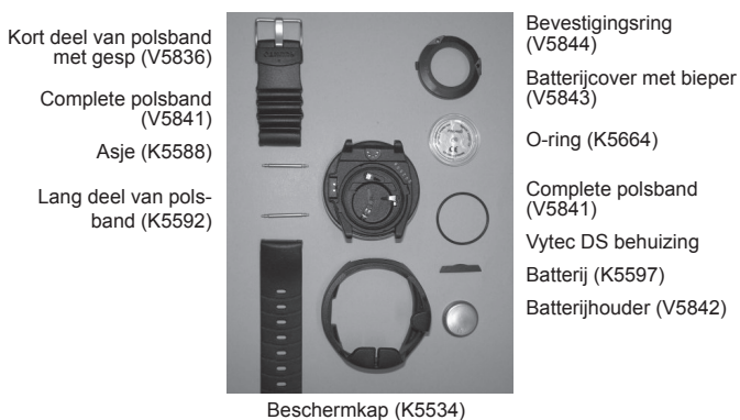
Fig. 5.1 Onderdelen. De code naast de benaming is de bestelcode.
