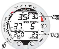
Fig. 3.18. Decompressieduik, binnen de decompressiezone. De twee naar elkaar wijzende driehoekjes vormen een zandloper. U bevindt u binnen de optimale decompressiezone op 3.5 m diepte en uw resterende opstijgtijd is minimaal 5 min. Door op de TIME knop te drukken kunt u het alternatieve display oproepen.
