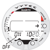
Fig. 4.32. Instellen van de wekker.
