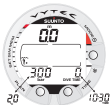
Fig. 3.3. Startup III. De Surface Mode of oppervlaktestand: De diepte en duiktijd zijn 0, de flesdruk is 300 bar. Door op de TIME knop te drukken activeert u de alternatieve displays met de temperatuur en de huidige tijd.
