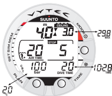
Fig. 3.14. Een Verplichte Veiligheidsstop. U wordt geacht om een Verplichte Veiligheidsstop te maken in het gebied tussen 6 en 3 meter diepte [20 ft en 10 ft]. Door het indrukken van de TIME knop kunt u het alternatieve display oproepen.
