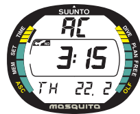
Abb. 2.3. Die Aktivierung des Wasserkontakts wird durch den Text "AC" dargestellt.
