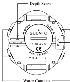
Abb. 2.2. Wasserkontakt und Drucksensor.
